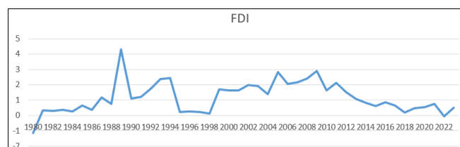
Fig 1: FDI
